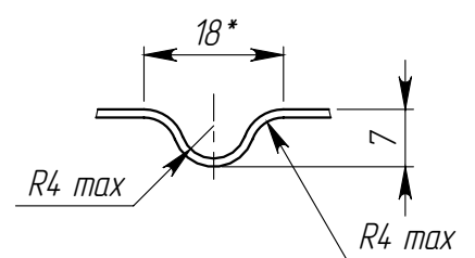
Вид 3 (1 : 1)
