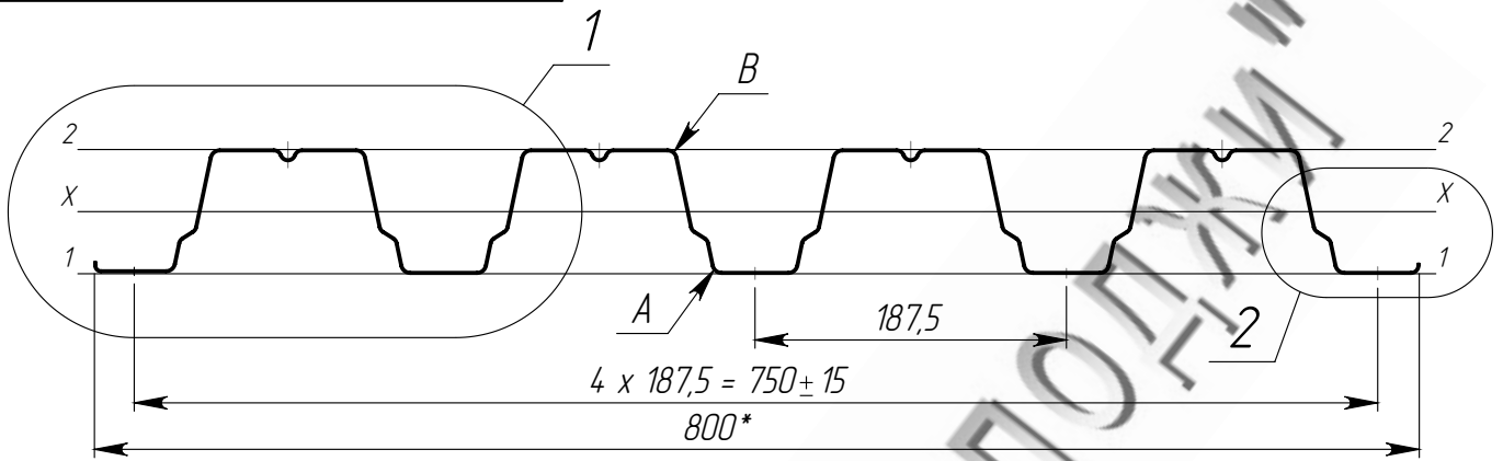
Вид 1 (1 : 2)
