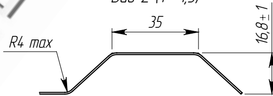
Вид 2 (1 : 1,5)
