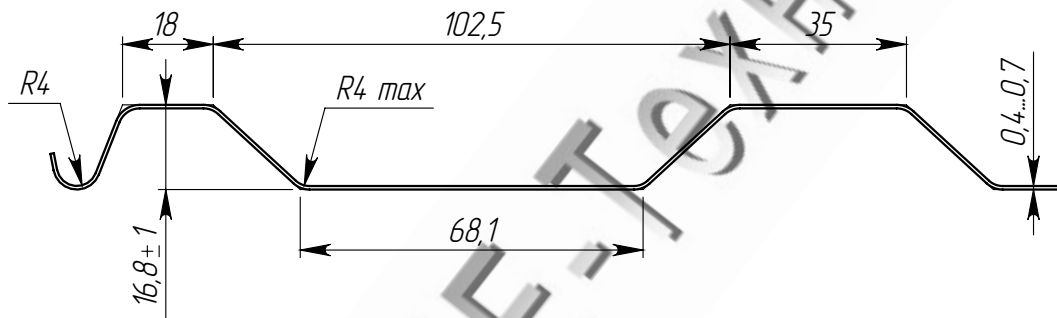
Вид 2 (1 : 1,5)
